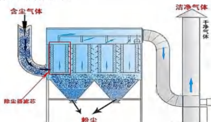
图4-2 布袋除尘器工作原理图
