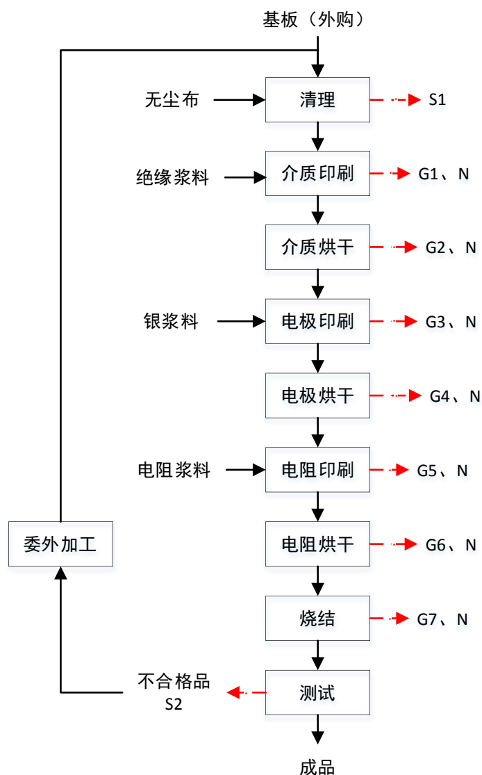
图 2-2 新能源汽车高压加热器工艺流程图
