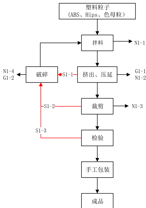
图 2-2 塑料板工艺流程图
