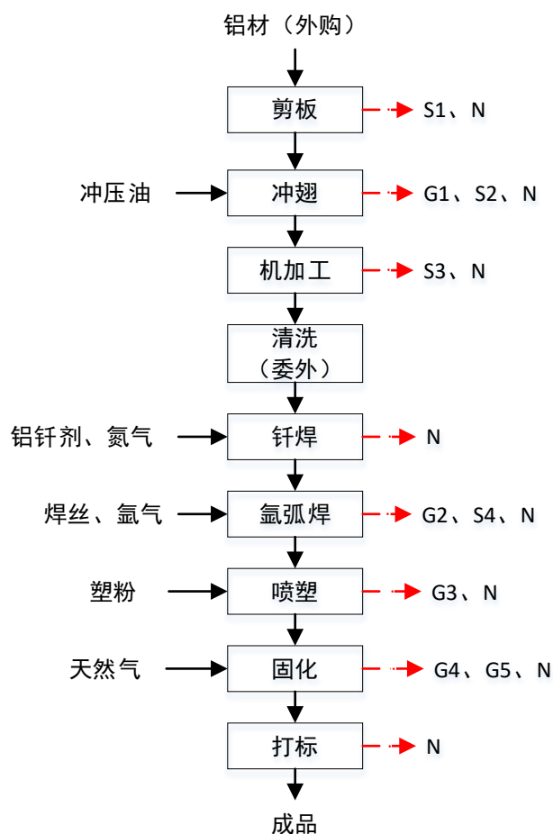
图 2-3 生产工艺流程图
