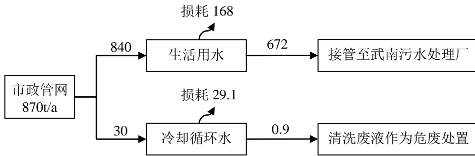
图 2-1 验收项目水平衡图 (t/a)
