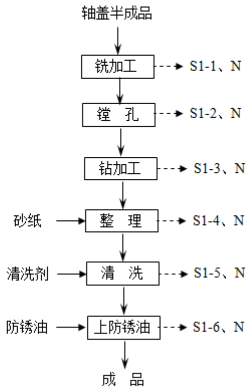
图 2-2 轴盖工艺流程图
