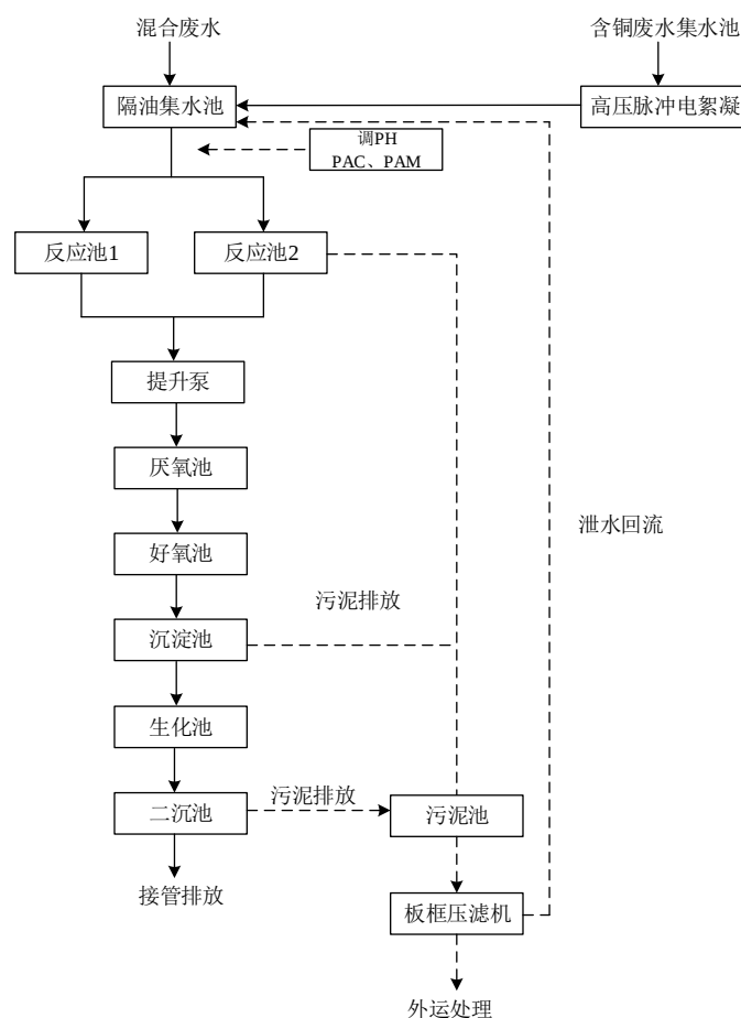
图 3-2 厂内污水处理站工艺流程图
