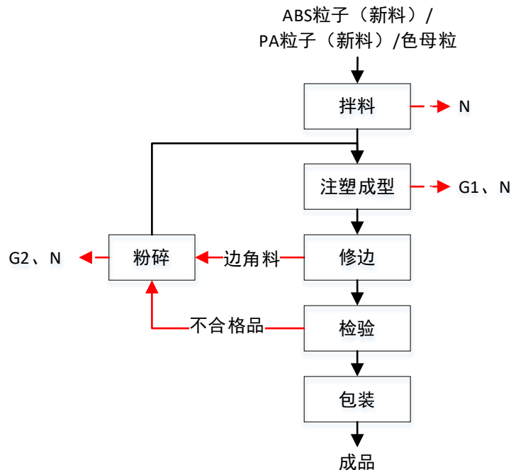
图 2-2 塑料制品生产工艺流程图（注：Gn：废气污染物；N：噪声）
